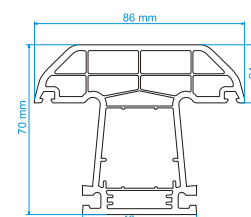
T profil UT 70 težina 1,420 kg/m
