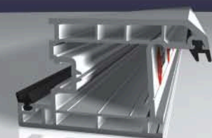
Krilo vrata unutrašnje UZK 60 težina 1,500 kg/m
