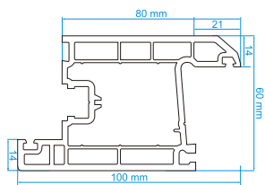
Krilo vrata unutrašnje UZK 60 težina 1,500 kg/m
