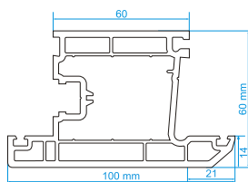
Krilo vrata spoljašnje UZKD 60 težina 1,600 kg/m
