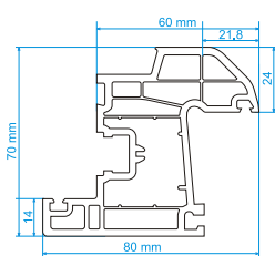
Krilo prozora UZ 70 težina 1,400 kg/m
