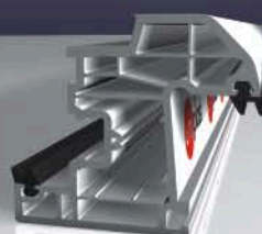
Krilo prozora UZ 70 težina 1,400 kg/m
