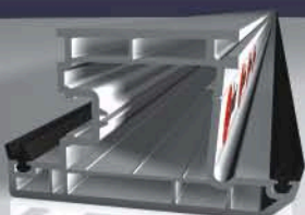
Krilo vrata spoljašnje UZKD 60 težina 1,600 kg/m
