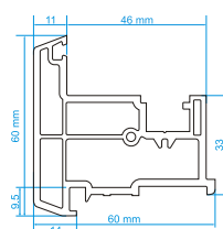
Reducir USZ 10 težina 0,900 kg/m
