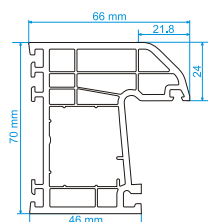
Štok profil UL 70 težina 1,250 kg/m
